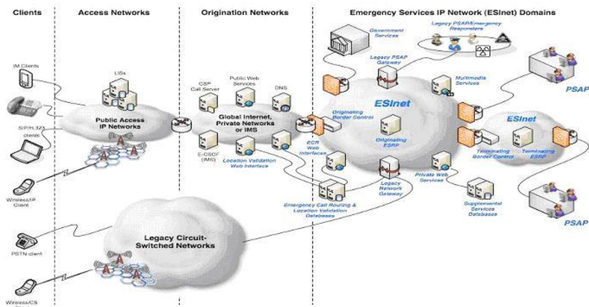
Abbildung: NG112 High Level Architecture nach EENA "Next Generation 112, Long Term Definition"
